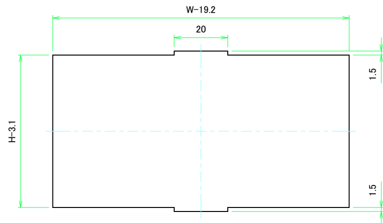
Wパネル1表面 / W Panel 1 Frontside
