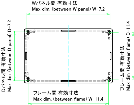
下カバー / Bottom cover
